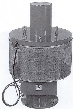
東部、岩子、柏崎、磯部に設置する 無志向型サイレン
